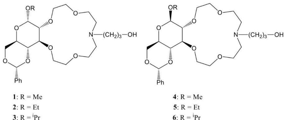
1. ábra: D-glükóz alapú lariat éterek
