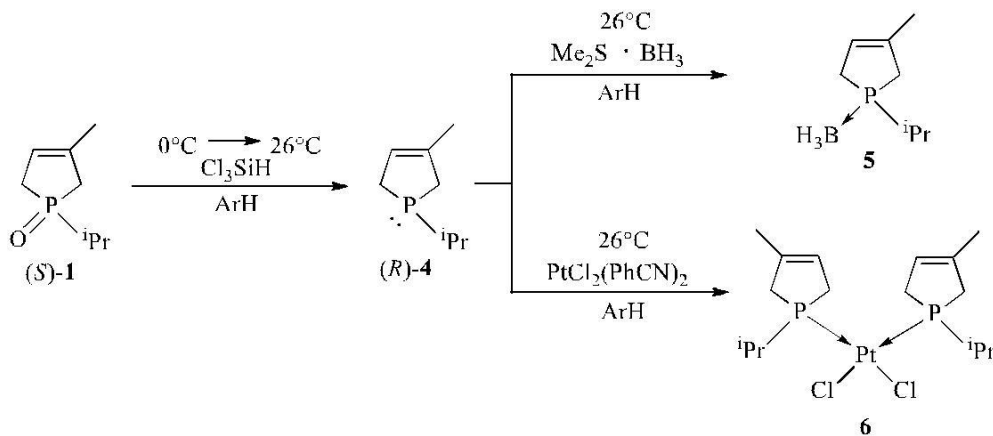
2. ábra: 1-izopropil-3-metil-3-foszfolén-borán és platina-komplexek (5 és 6)
