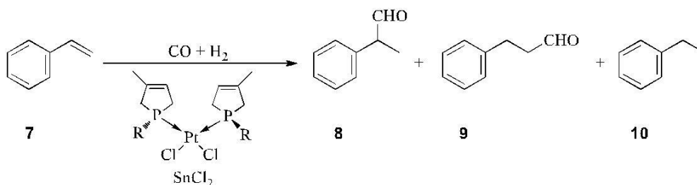
3. ábra: Szirol (7) hidroformilezése
