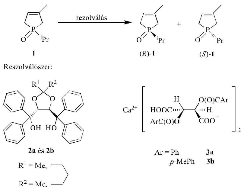
1. ábra: 1-Izopropil-3-metil-3-foszfolén-1-oxid (1) rezolválása
